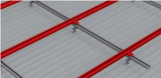
Illustration du procédé K2 SOLIDRAIL SOLARFASTENER PLAQUES NERVURÉES (DROM) (cas de la configuration B avec deux couches de rails)
