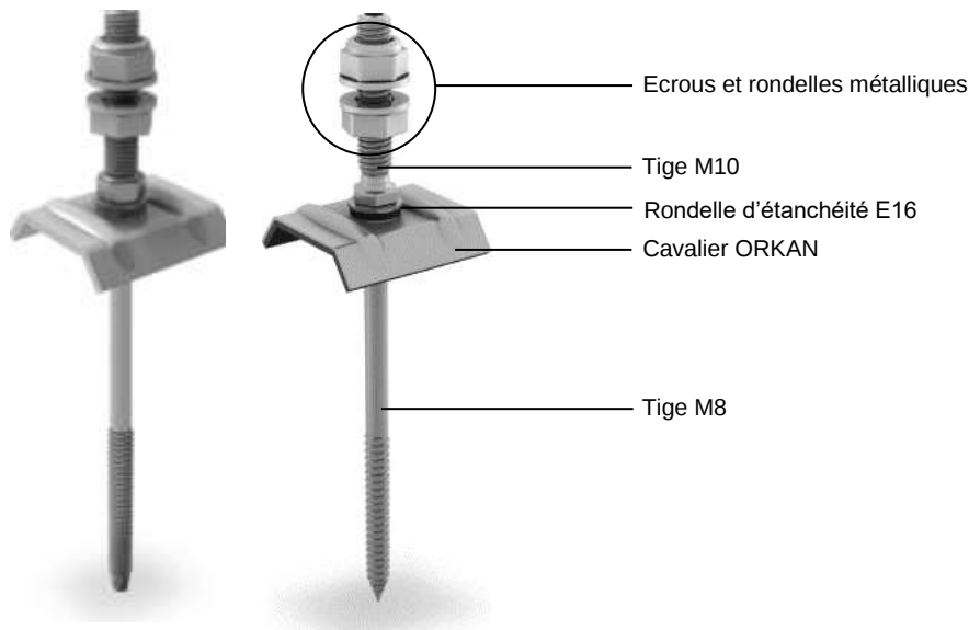
Vis de fixation pour panneaux solaires : (gauche) pour pannes en acier ; (droite) pour pannes en bois
